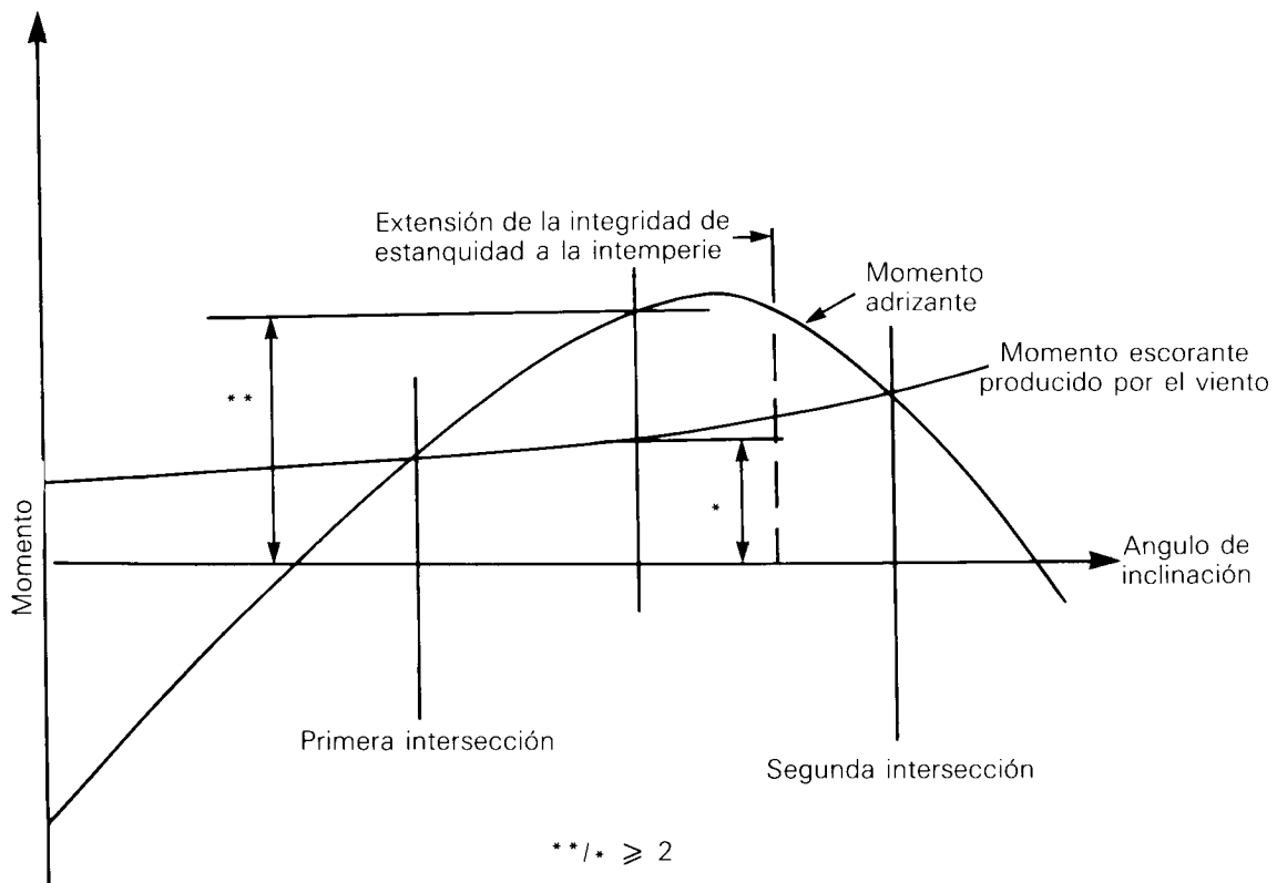
Figura 3-2 – Curvas de momentos adrizantes y de momentos escorantes producidos por el viento
