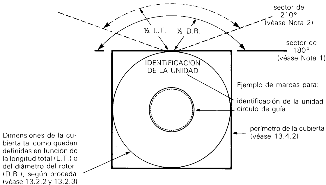
Figura 13-1 – Ejemplo de disposición de una cubierta para helicópteros
