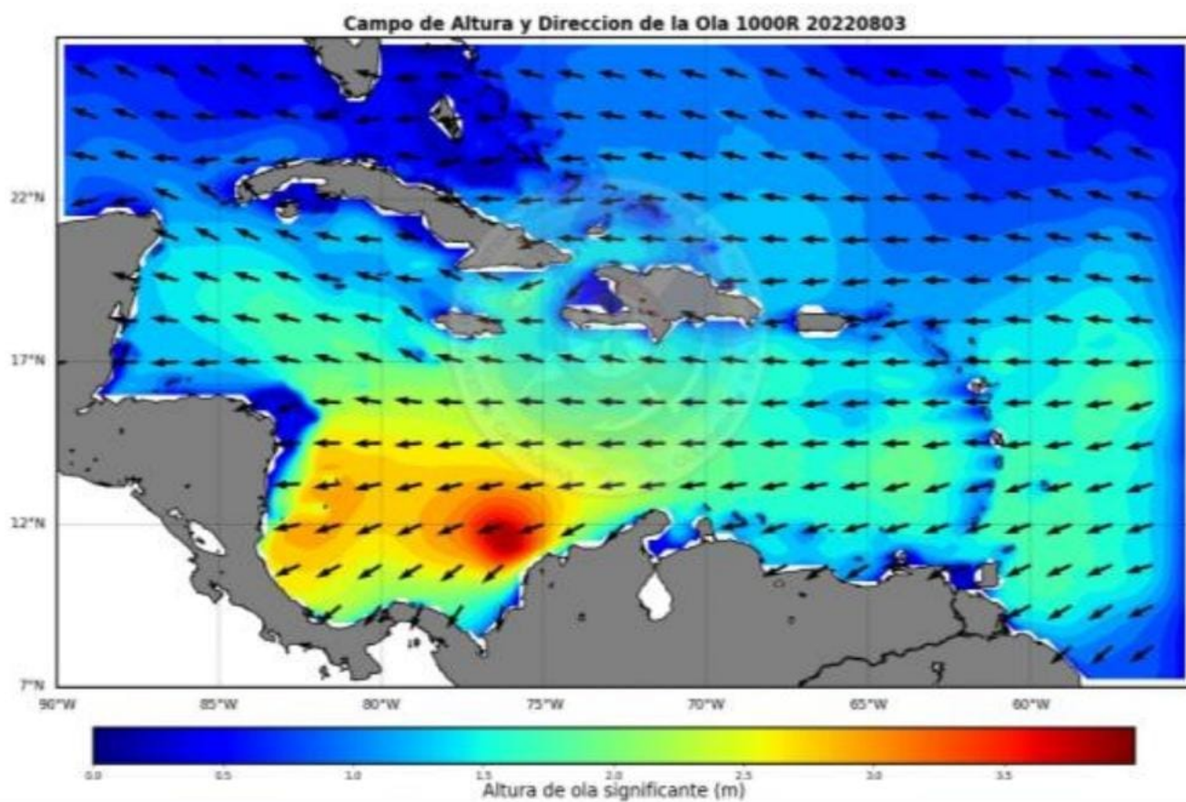
Figura 2. Pronóstico de altura significativa y dirección predominante del oleaje Mar Caribe para las 1000R del 03-08-2022. Fuente: modelo Wave Watch III – CIOH.
