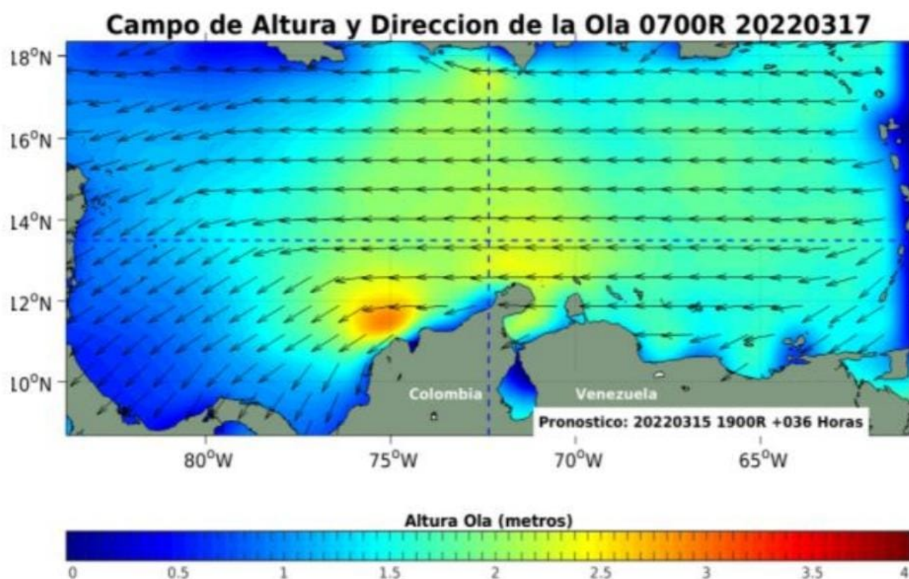
Figura 2. Pronóstico de altura significativa y dirección predominante del oleaje Mar Caribe para las 0700R del 17-03-2022. Fuente: modelo CaribWam – CIOH.
